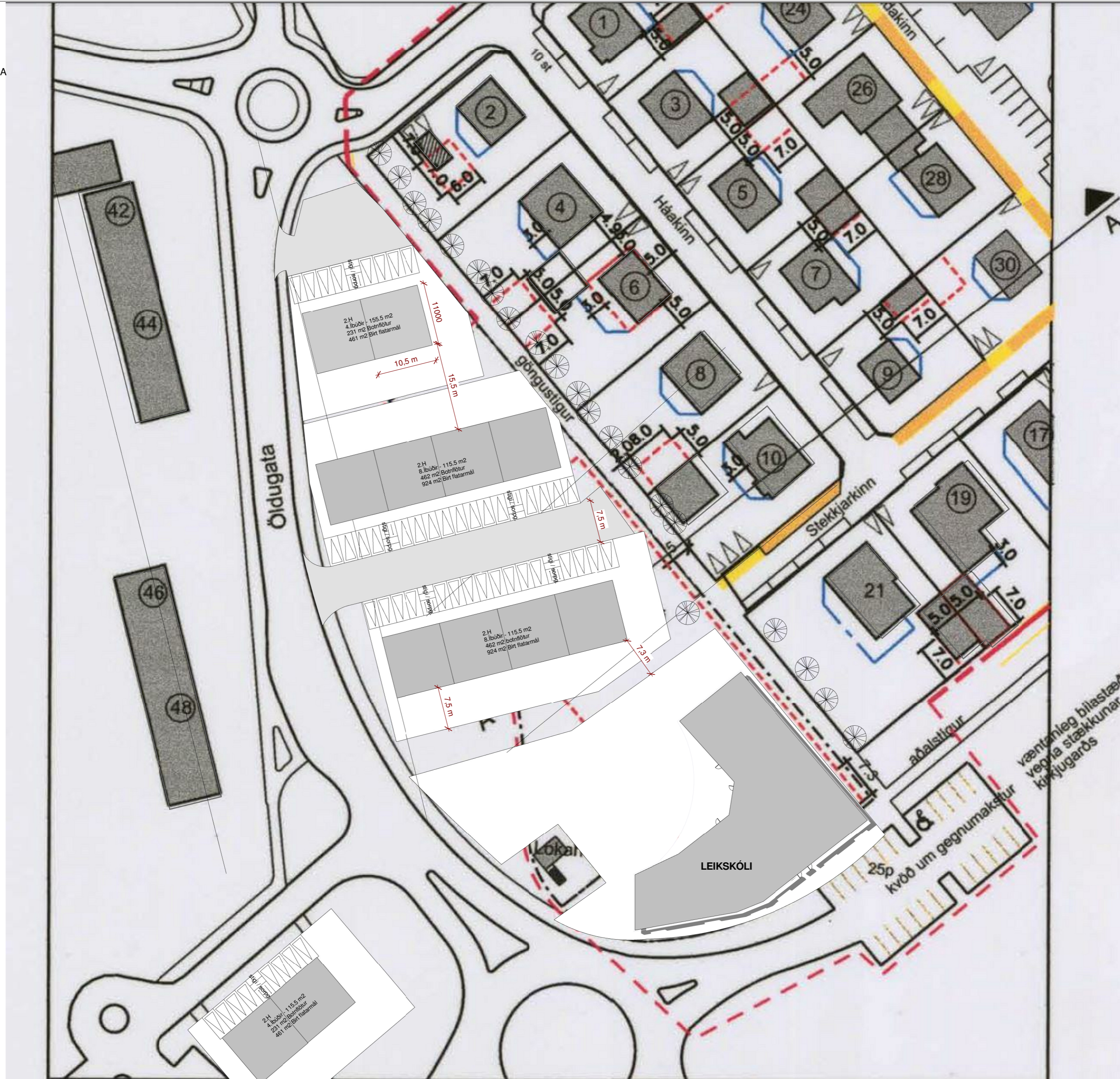
AFSTÖÐUMYND 1 : 500
